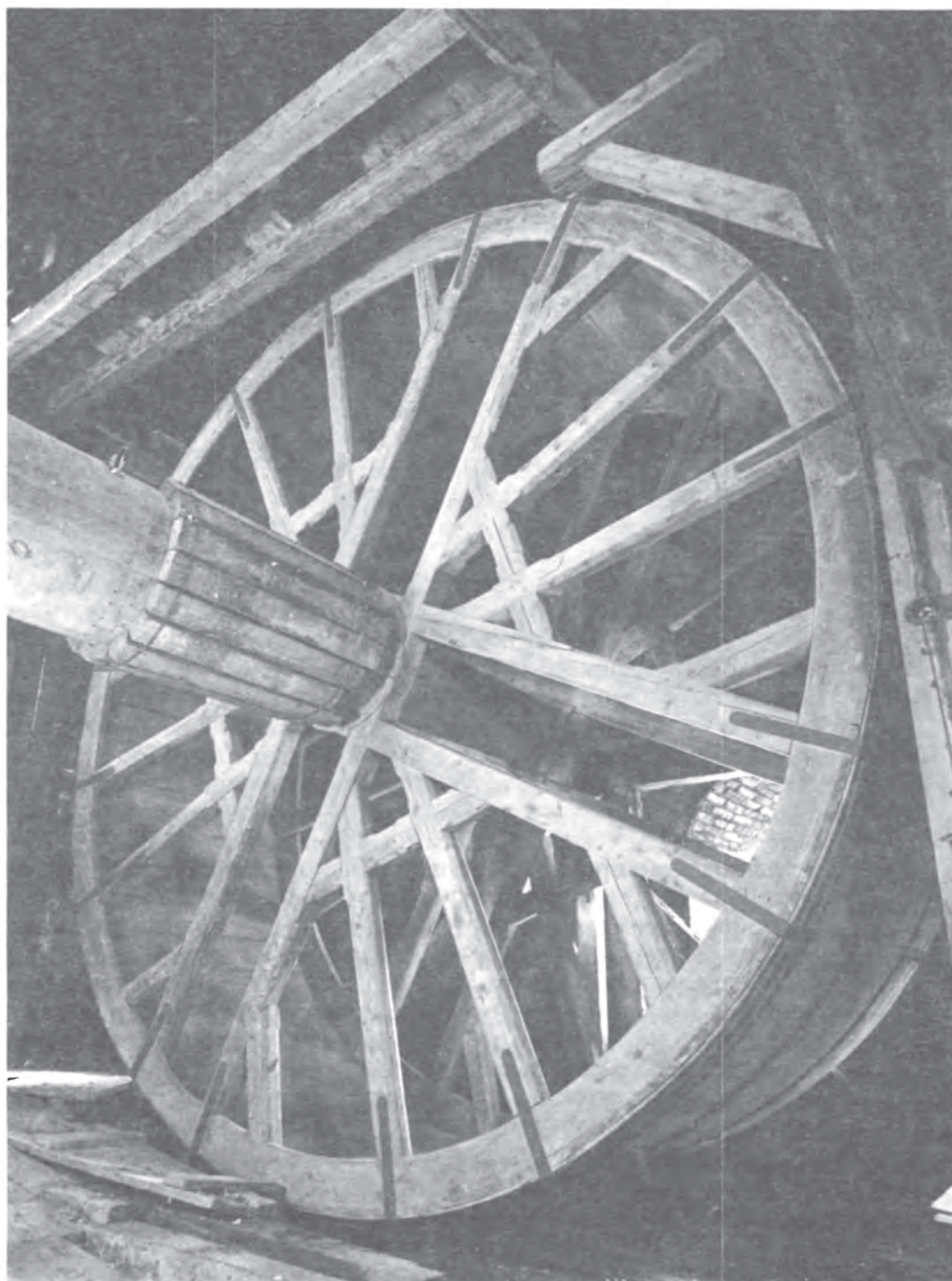
Машины и зубчатые передачи из дерева. Это огромное колесо горизонтального ворота было клеткой, которую приводили в движение помещавшиеся внутри нее три человека. Мюнхен. Немецкий музей, собрание фотоматериалов.
