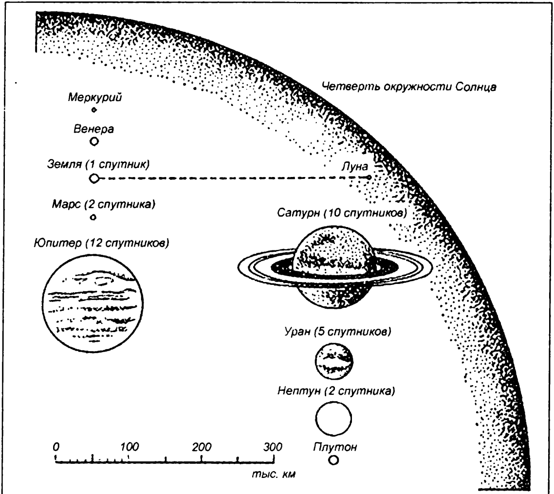
Сравнительные размеры планет и Солнца
